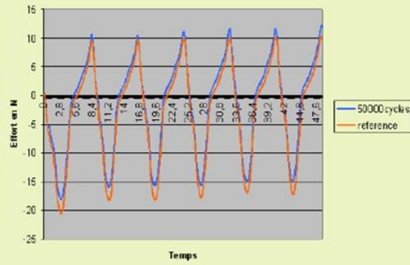
Comparaison de palmes neuves et de palmes après 50 000 cycles de palmages
