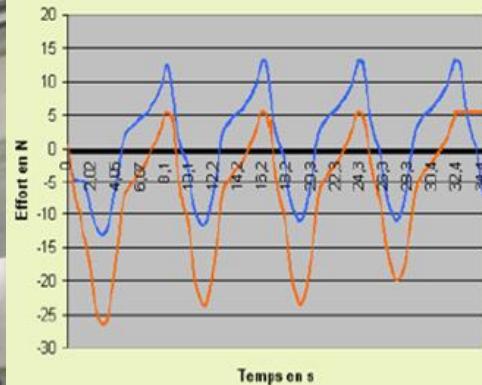
Comparaison de palmes neuves et de palmes après 50 000 cycles de palmages
